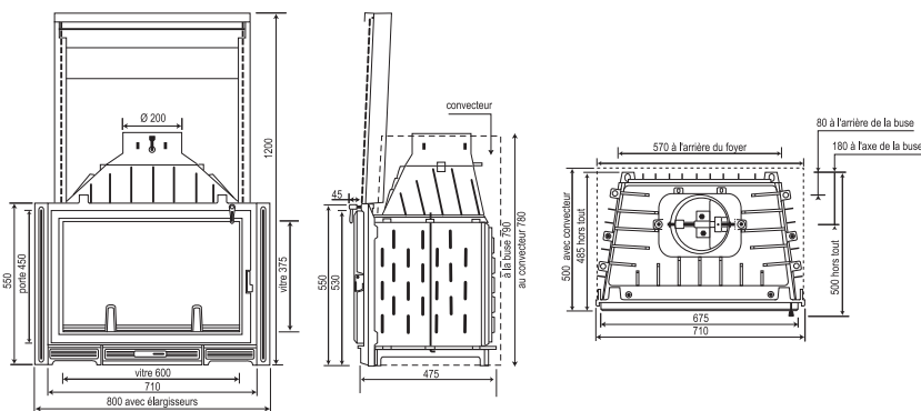
Façade 80 cm
