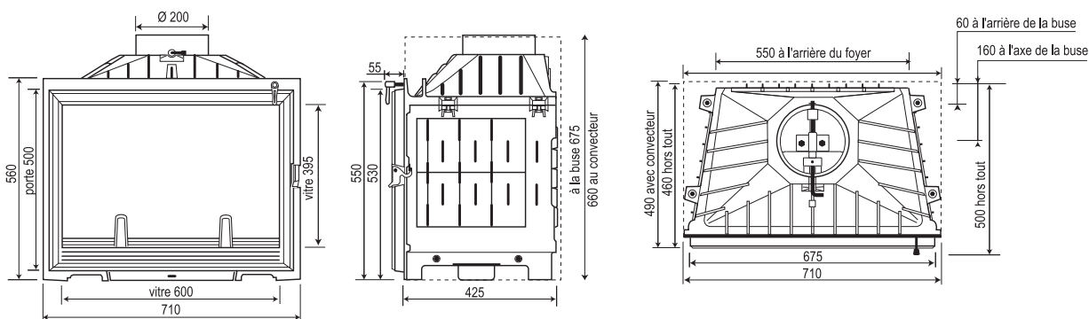
convecteur
